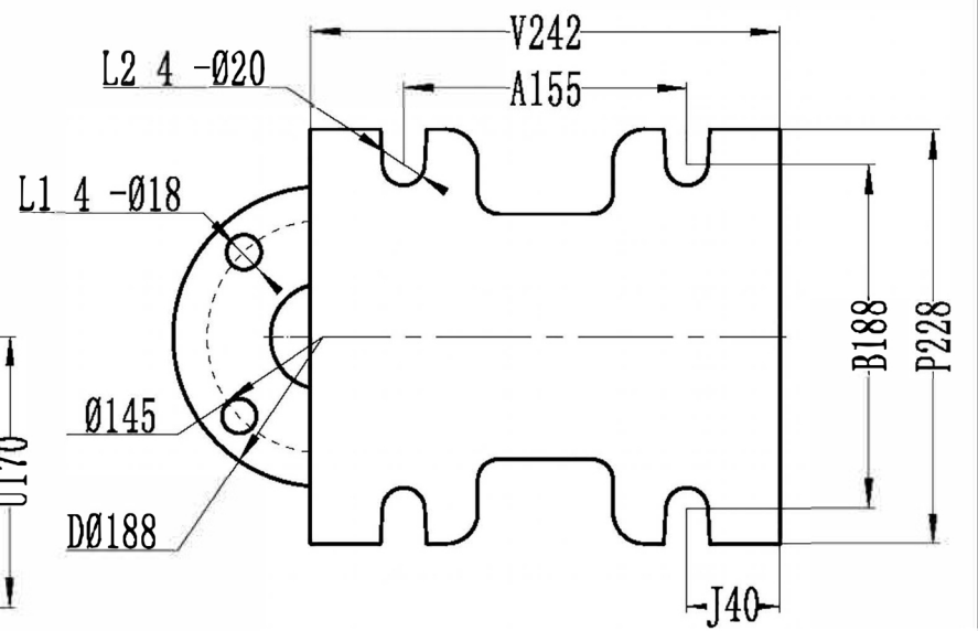
Auto-coupling DN65 PN10
