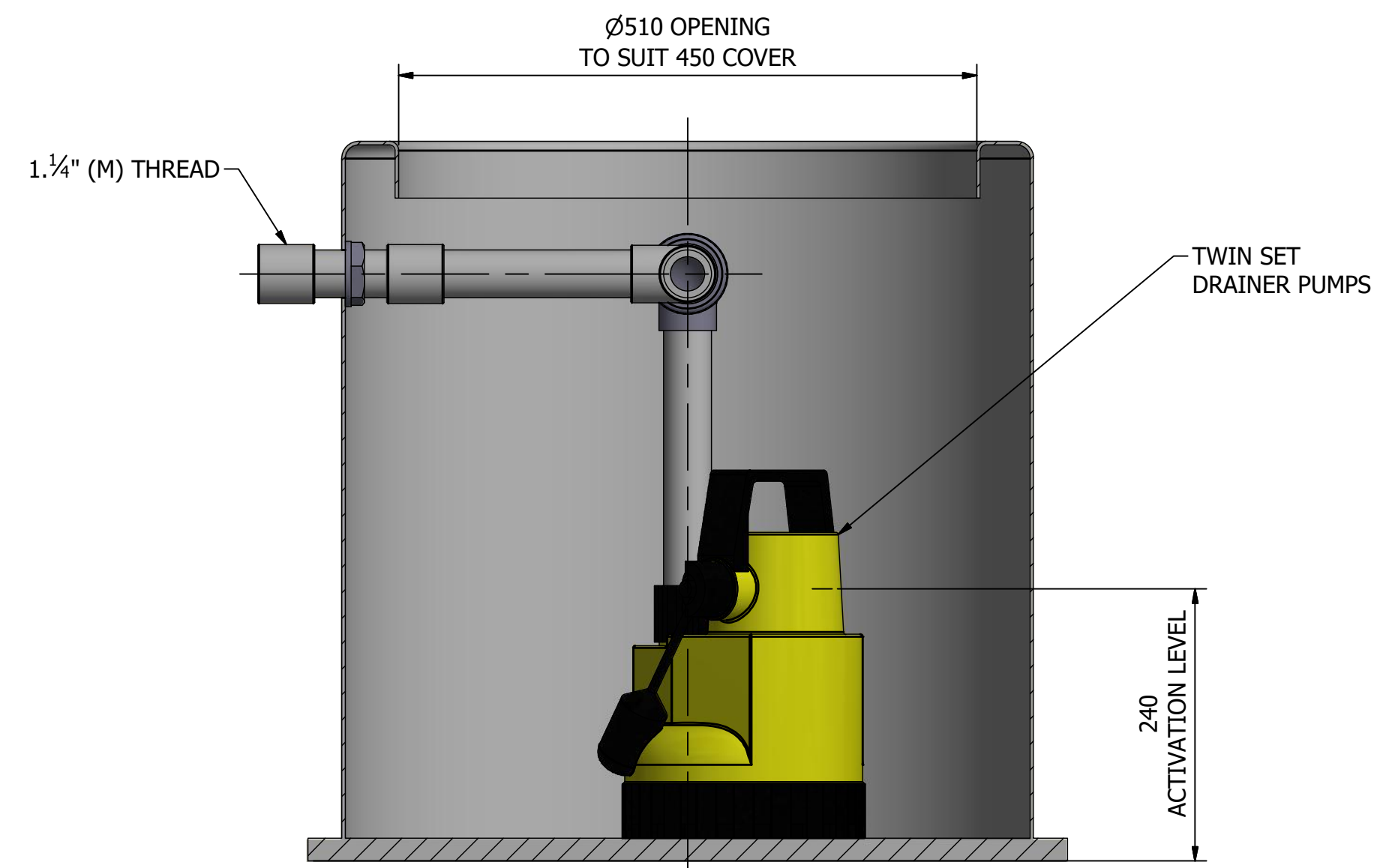
SECTION A-A SCALE 1:5
