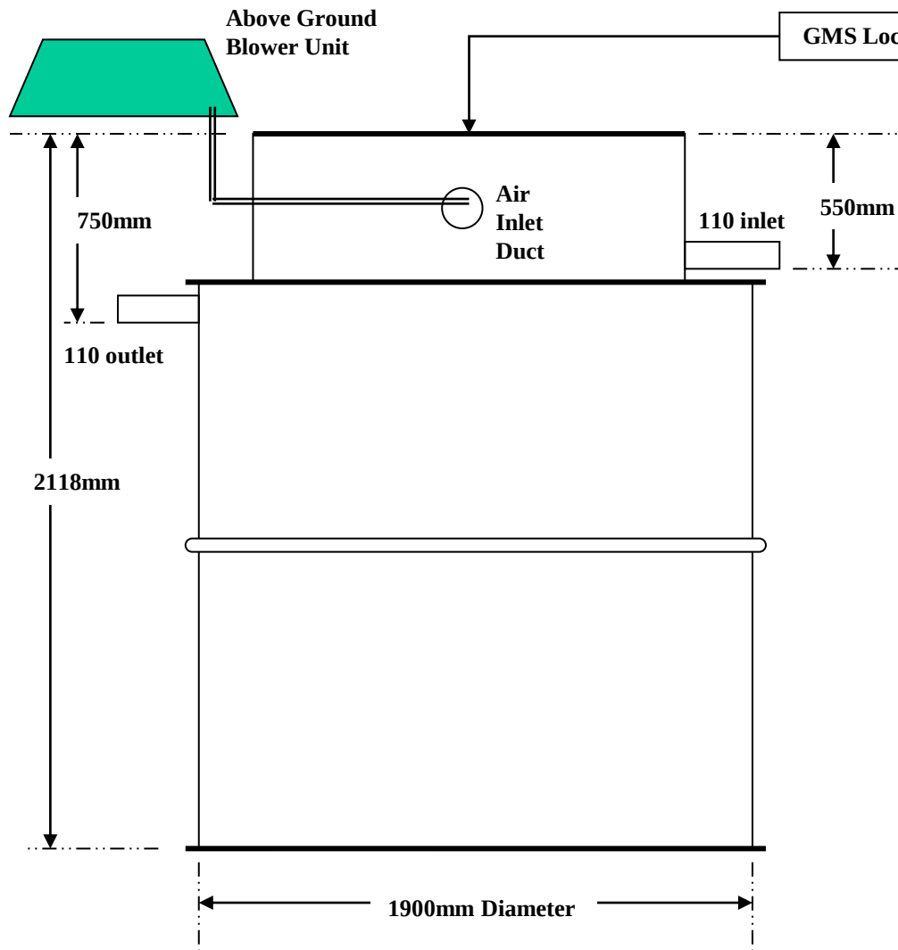
ELEVATION
